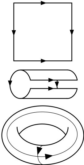
Po utożsamieniu przeciwległych boków kwadratu otrzymujemy torus.
