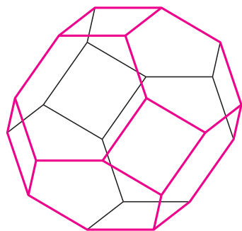
Czternastościan archimedesowy
