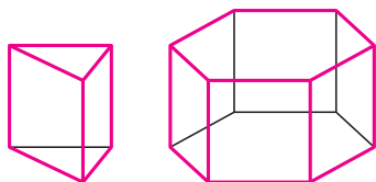
Wypełniająca przestrzeń graniastosłupy archimedesowe (ten z prawej znany jest w budownictwie drogowym jako trylinka)
